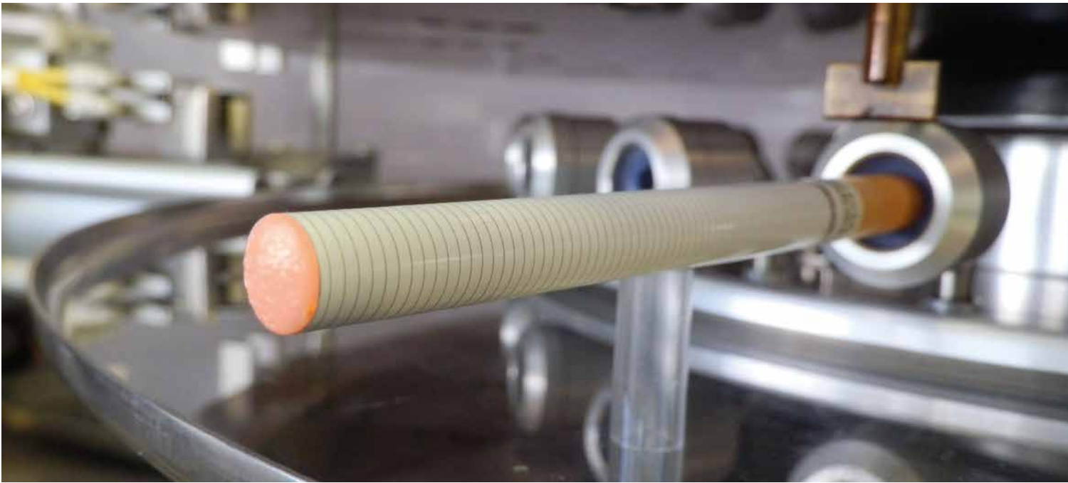
E-Zigarette in einer speziellen Abrauchmaschine am CVUA Sigmaringen für die Prüfung auf Schadstoffe
